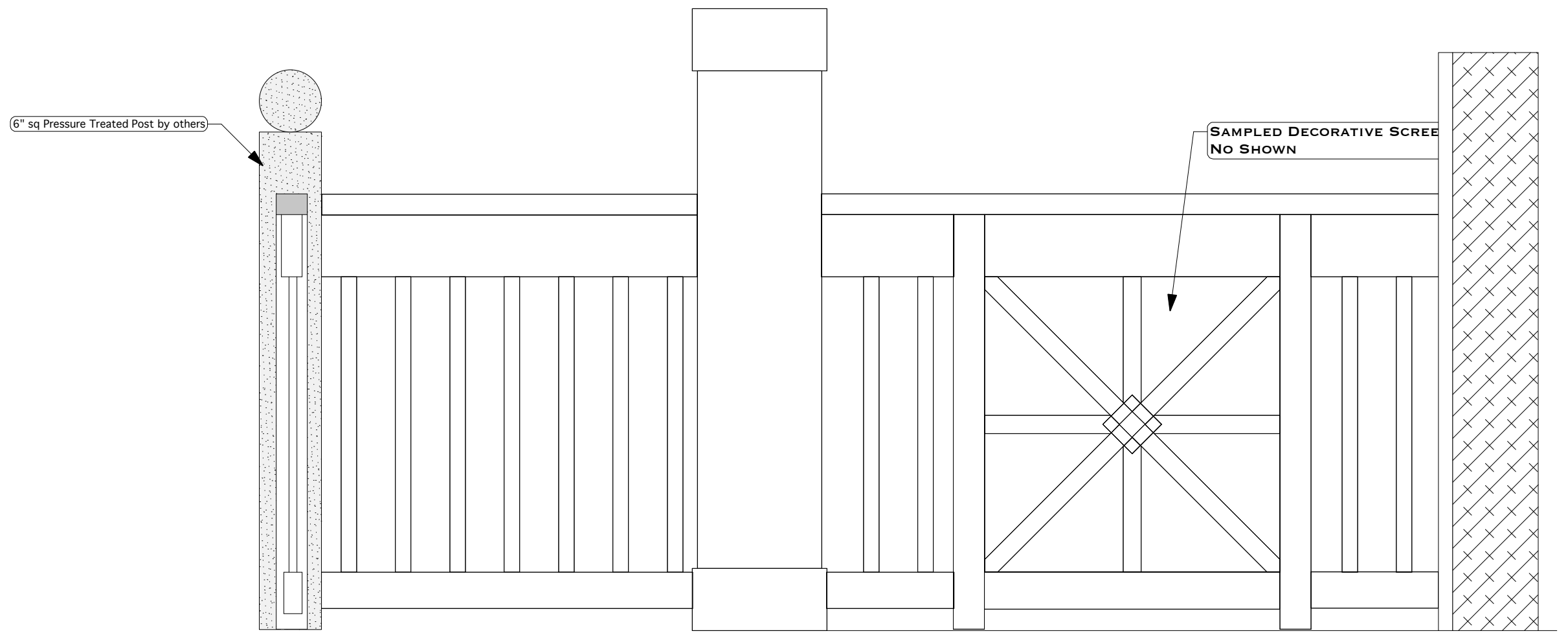
SIDE VIEW PATIO SCALE: 1" = 1'-0"
